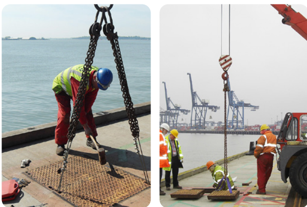
Arbeitsintensive Vorgehensweise bei der Entfernung der bestehenden Abdeckungen
