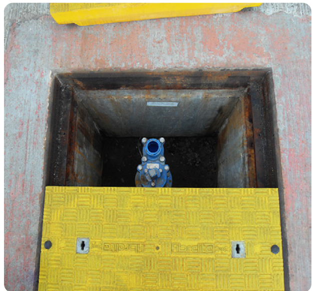
Früher mussten zwei extrem schwere Stahlabdeckungen entfernt werden, um an den Hydranten für die Trinkwasserversorgung zu gelangen. Dank der Faserverbundabdeckung gehört das der Vergangenheit an.
